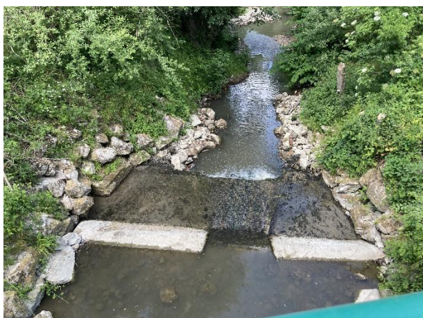
Seuil jaugeur de la station hydrométrique de la Biesme au Claon avant travaux, vu du pont de la RD 84. Dénivelé amont-aval de 80 cm. Malgré l'échancrure centrale sur la partie amont du seuil béton le radier aval est infranchissable et une chute demeure en aval du radier.
